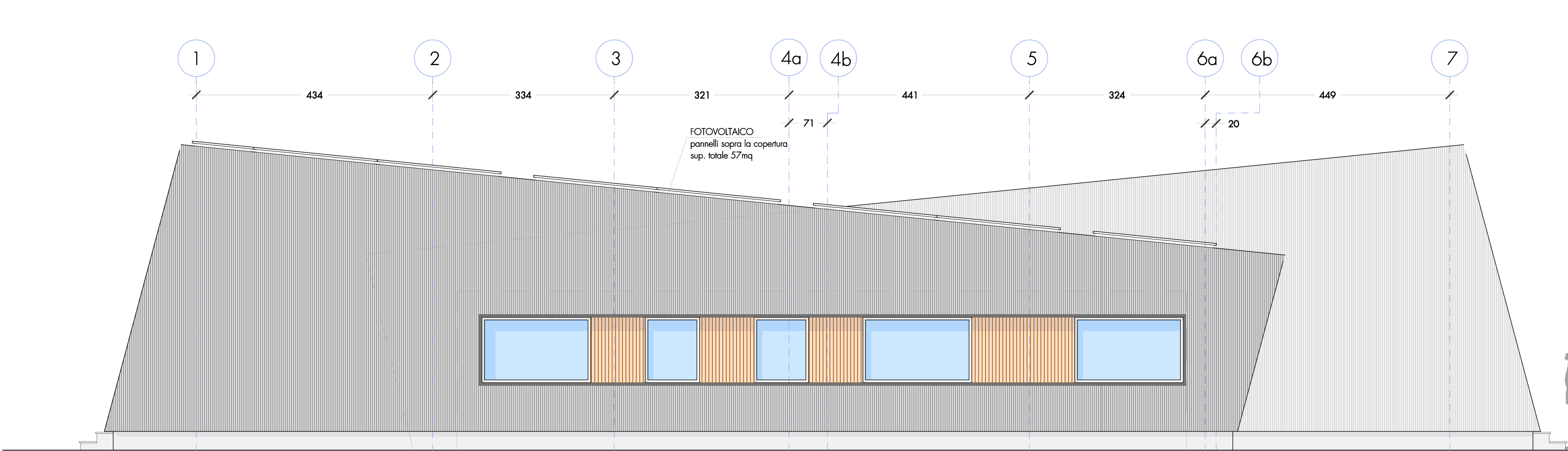
PROSPETTO OVEST Scala 1:50
